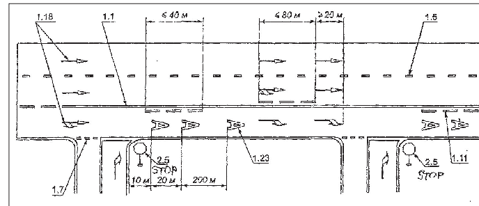
Вот так должна выглядеть разметка у въезда-выезда согласно ГОСТУ Р52289-2004. Источник: Приказ Ростехрегулирования от 15.12.2004 № 120-ст.
