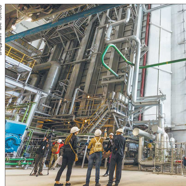
Оборудование Верхнетагильской электростанции поражает своими масштабами. На фото — газовая турбина с генератором производства Siemens. Её мощность — 305,9 МВт
