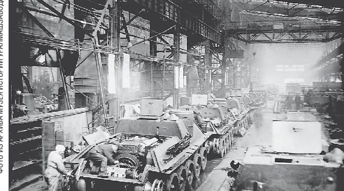
Поточная линия сборки самоходок в цехе 1 Уралмашзавода
