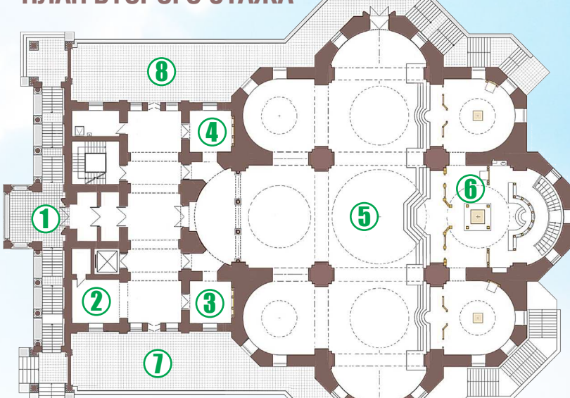
1. паперть; 2. свечная лавка; 3, 4. часовня; 5. храм; 6. алтарь; 7, 8. гупльбище.
