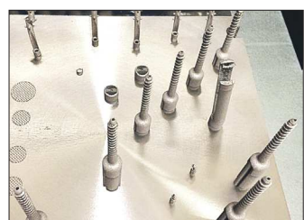
Экспериментальные уральские импланты – челюстной (на фото слева) и фаланги пальцев, внешне напоминающие шурупы (справа). Внутри у искусственных костей видна пористая структура
