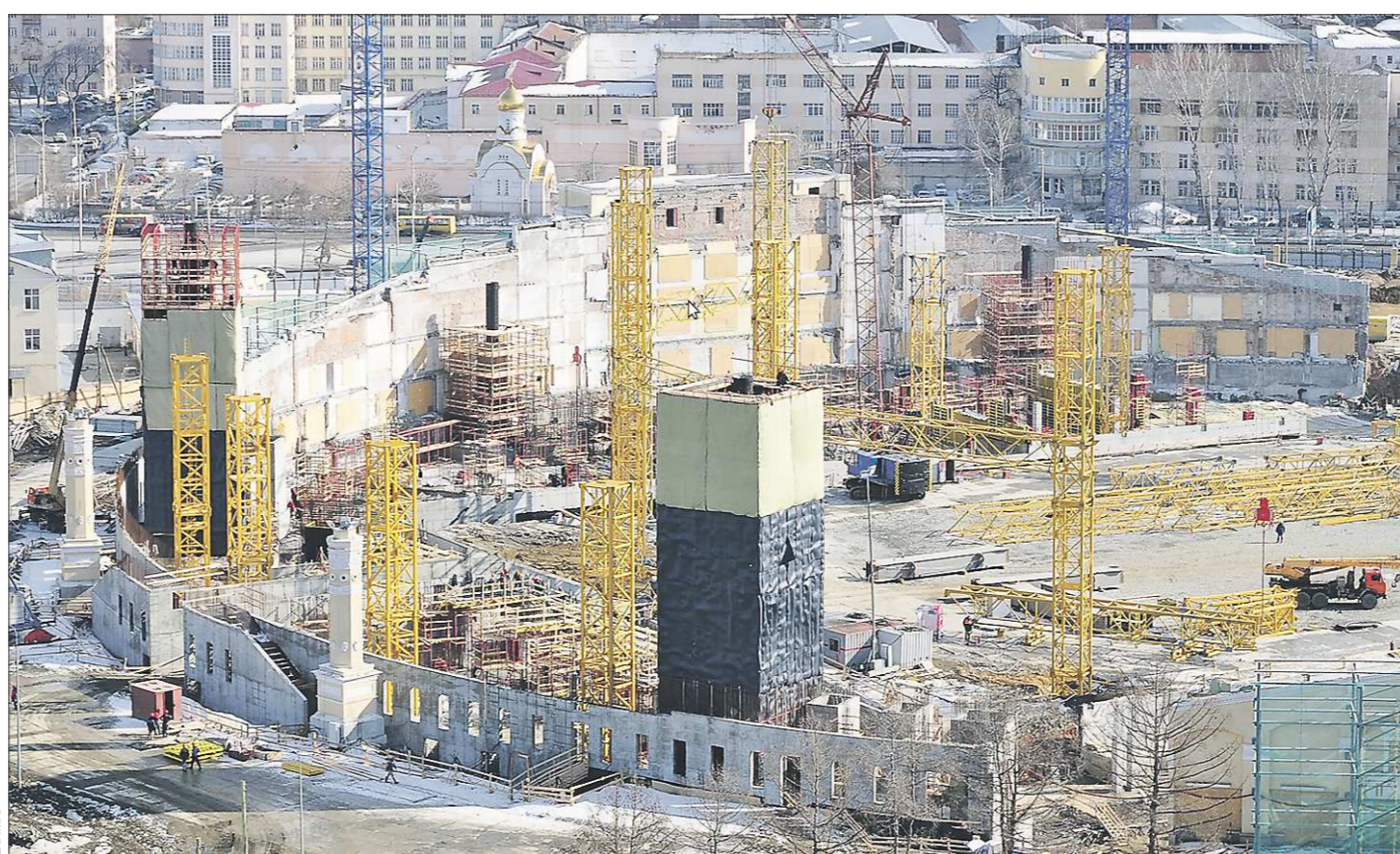
Пилоны — чёрные трубы диаметром три метра, на которые будет опираться навес Центрального стадиона, закрывающий все зрительские места
