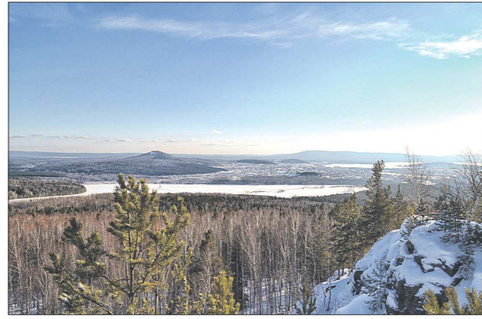
Где теперь раки зимуют? Из Черноисточинского пруда они ушли ещё восемь лет назад. Это говорит об ухудшении качества воды
