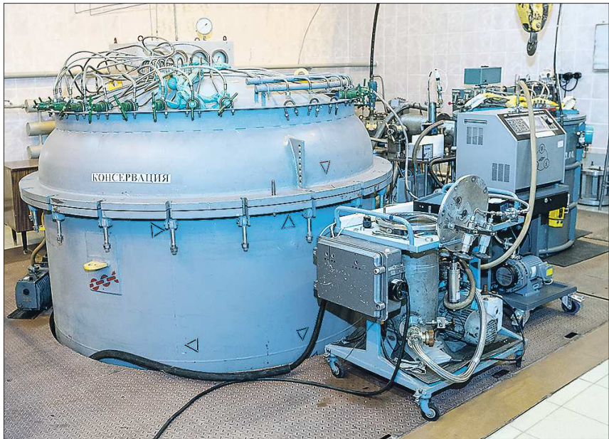
В этой камере проходят вакуумные испытания микродвигателей НИИМАСШа, часть оборудования изготовлена на самом предприятии
