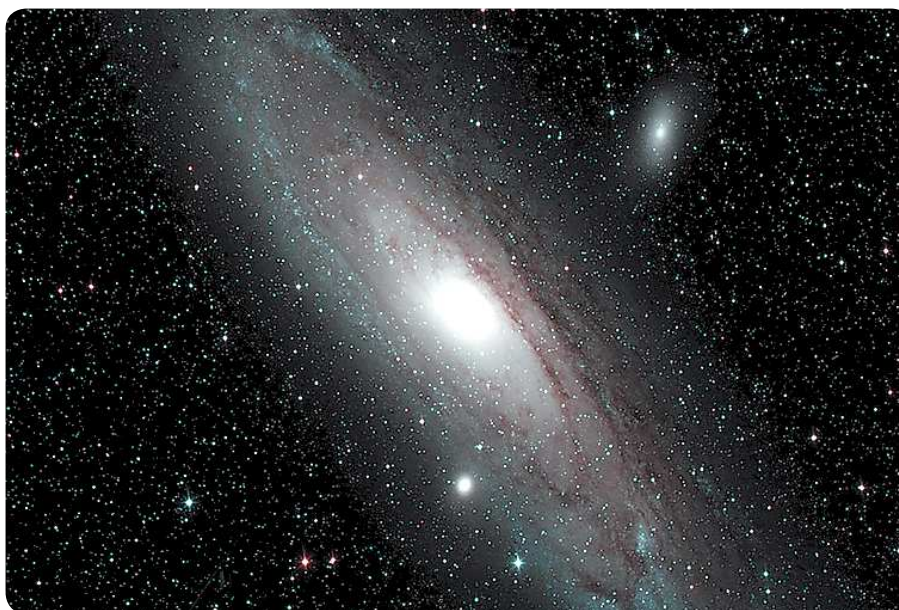
Туманность Андромеды
