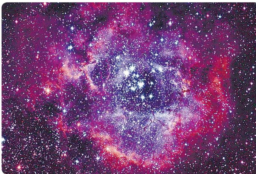
Туманность Розетка
