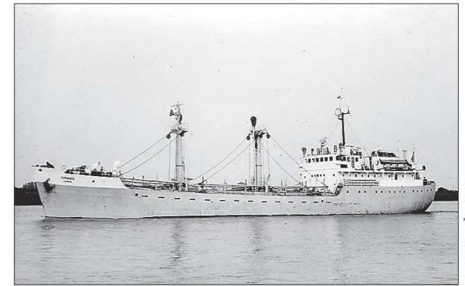
Длина этого судна составляла 70 метров, ширина — 10. Масса — 1072 тонны
