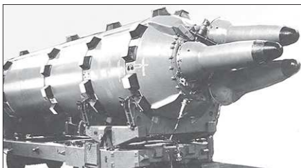
Длина ракеты Р-27 составляла 8 метров 89 сантиметров, а вес — 14 тонн 200 кг
