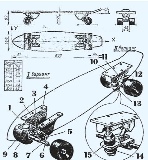
СХЕМА ИЗ ЖУРНАЛА «ЮНЫЙ ТЕХНИК» 6/1978
