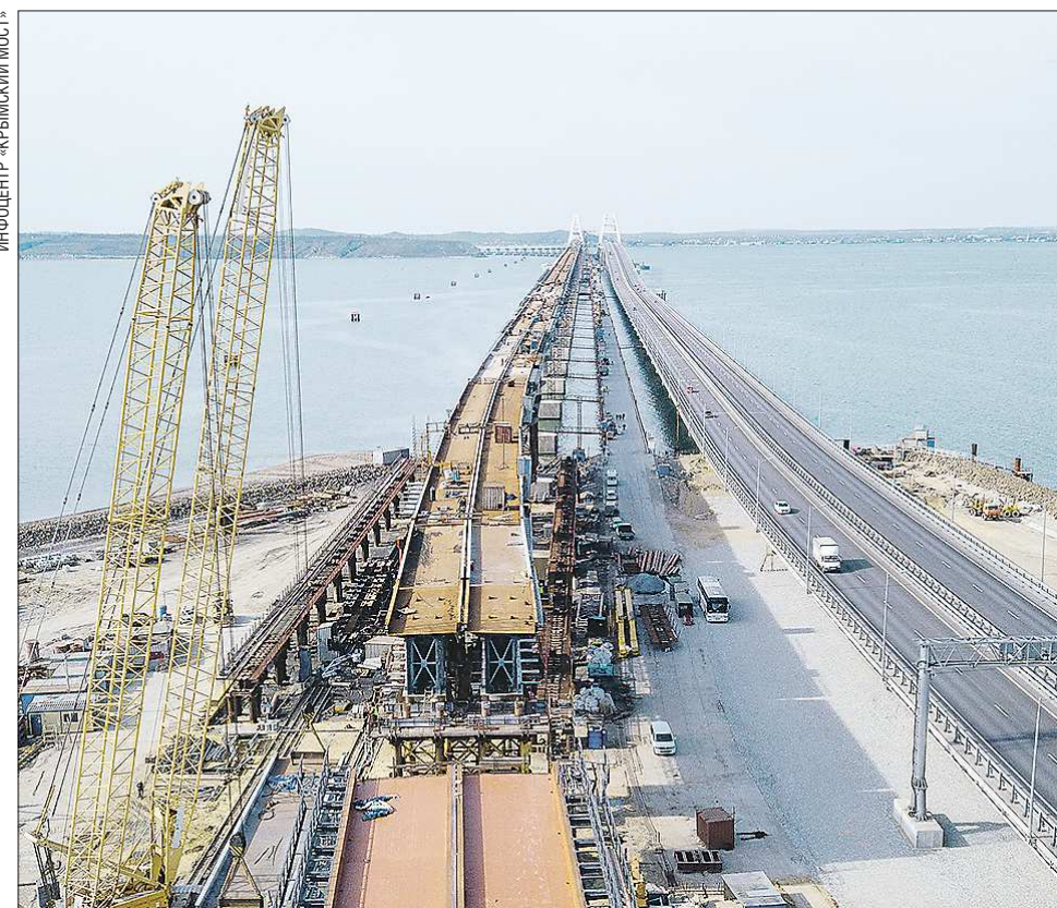
Крымский мост является самым крупным в России - его протяжённость составляет 19 километров
