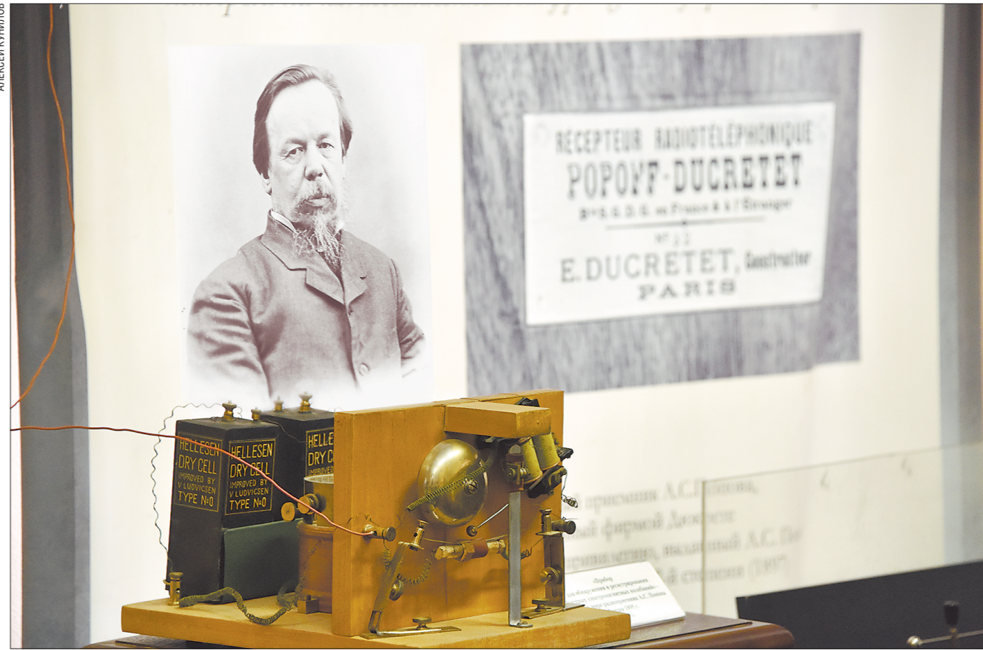
На фото - макет первого радиоприёмника, собранного Александром Поповым. Именно с него началась эра радио. Он выставлен в Екатеринбургском музее радио имени Попова
