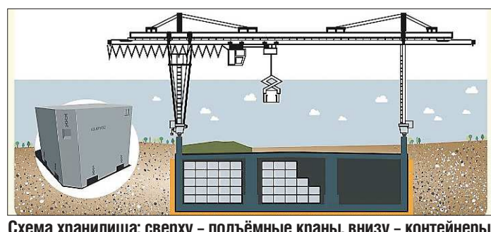
Схема хранилища: сверху — подъемные краны, внизу — контейнеры
