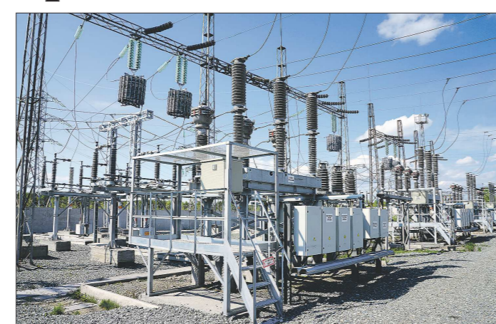
Подстанция «Ферросплав» в день пуска
