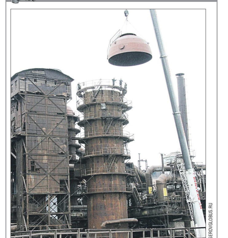
На Серовском металлургическом заводе идёт реконструкция, пишет газета «Глобус». На одну из доменных печей установили три 12-тонных купола. Вместе с подъёмом на высоту в 30 метров процесс занял всего два часа - благодаря специальному прихватуем из Екатеринбурга мощному автокрану получился быстро. Установка купола таким способом производится второй раз за всю историю металлургического завода. Обычно купол поднимали по частям и уже вверху сваривали. Доменную печь планируют запустить во второй половине 2015 года
