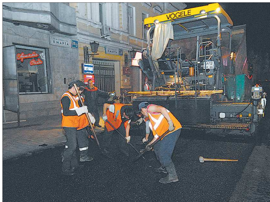
Без ручного труда при ремонте дорог всё же не обойтись. Когда на объекте встречается люк, на помощь самой современной техники приходят специалисты с лопатами
