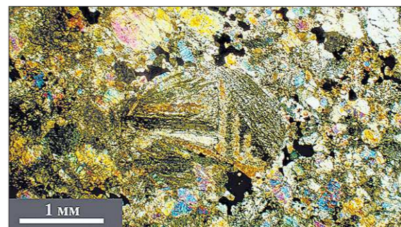
На увеличенном под микроскопом образце хорошо видны игольчатые тела. Это и есть хондры, из-за которых метеориты каменного типа называются «хондритами»
