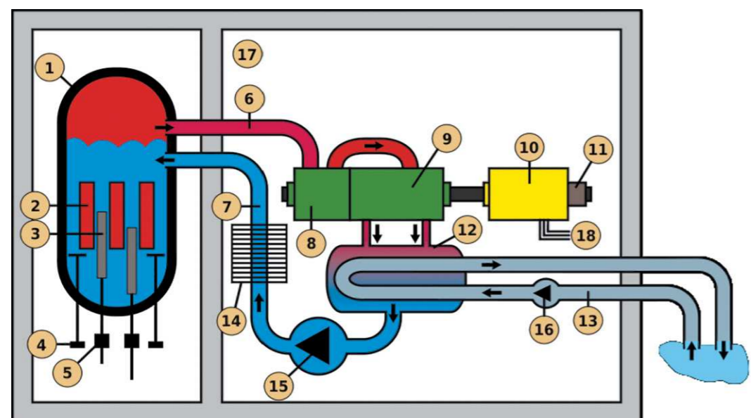
Схема работы ядерного реактора кипящего типа, какие установлены на «Фукусиме»
