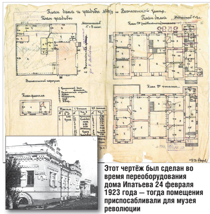
Этот чертёж был сделан во время переоборудования дома Ипатьева 24 февраля 1923 года — тогда помещения приспосабливали для музея революции
