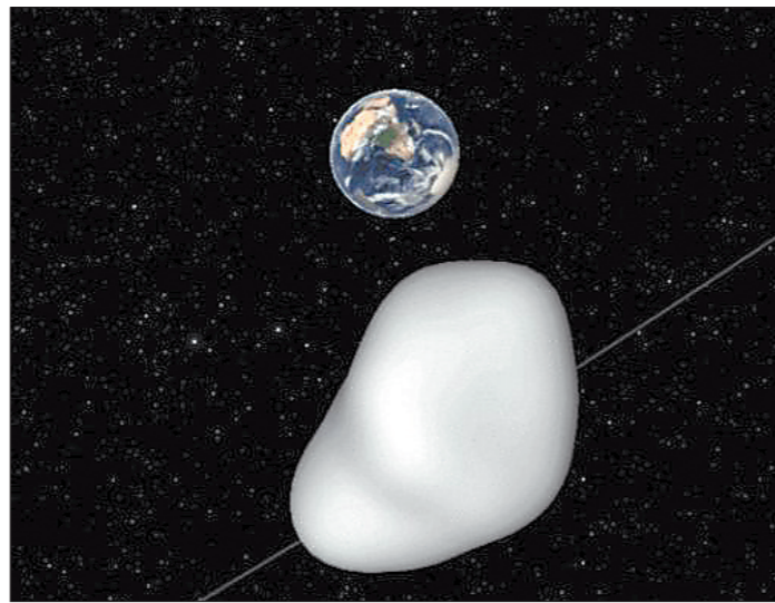
Траектория полета астероида 2012 TC4 прошла по касательной линии к орбите Земли
