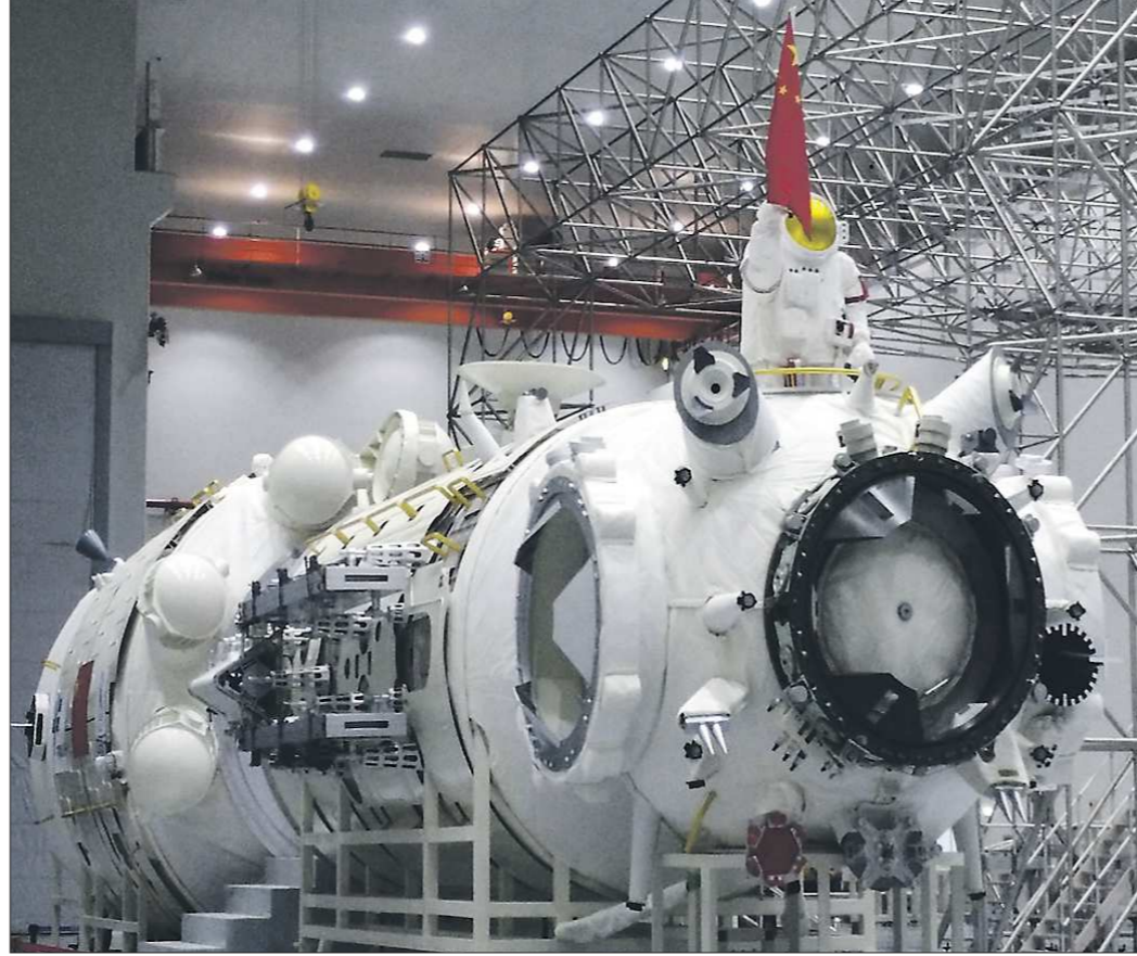
Прототип базового модуля «Тяньхэ» в сборочном цехе космодрома Вэньчан
