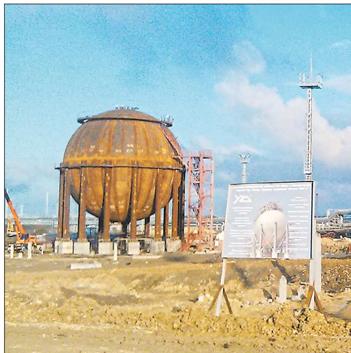
Шаровые резервуары на площадке в порту Тамань
